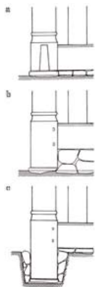
Tegning c er av en jordgravet stolpe. Tegningene a og b er av staver på fundament over bakken. J. H. Jensenius.
